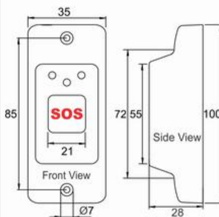
10 ~ 30 Volt DC IP67 'NC' Switch SOS Button
