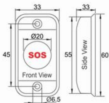
10 ~ 30 Volt DC IP67 'NC' Switch SOS Button
